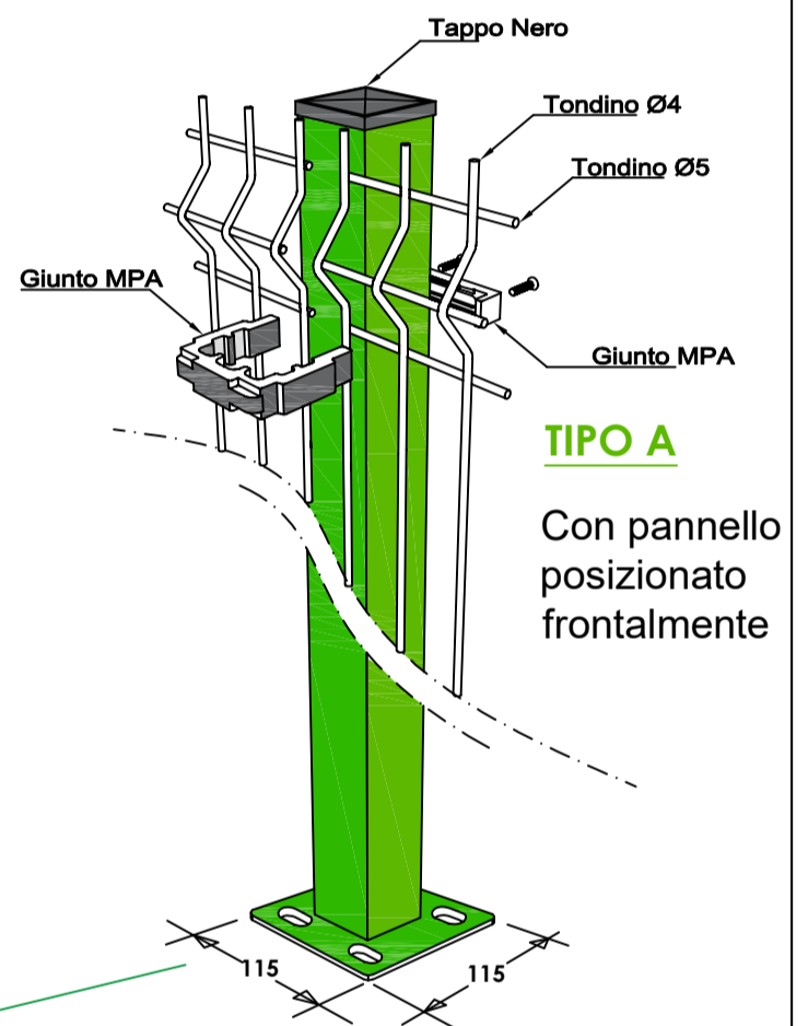
PIASTRA 115x115x8 DOTATA DI N° 04 ASOLE 13x28 mm
